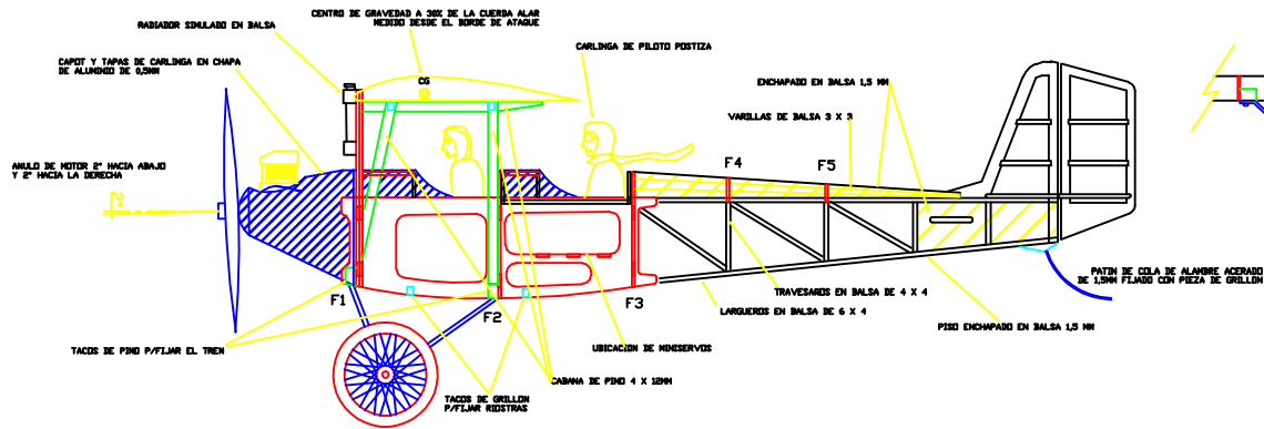
GRUPO DE COLA EN Balsa DE 4 MM DE ESPESOR
